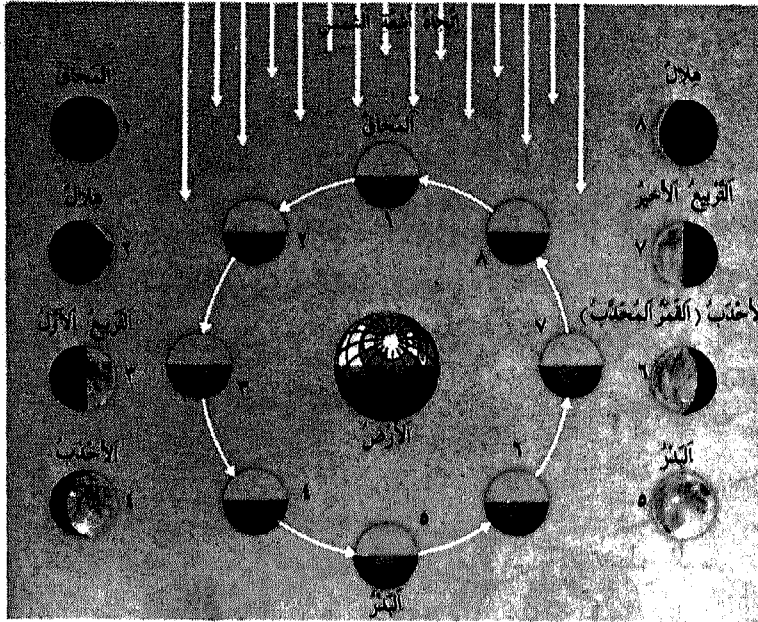
شكل ( 3 ) اشكال القمر: ابتداءً من حالة المحاق رقم ( 1 ) الى البدر رقم ( 5 ) ثم يعود الى الحالة الأولية بعد أن يمر بأشكال ما بينهما.
